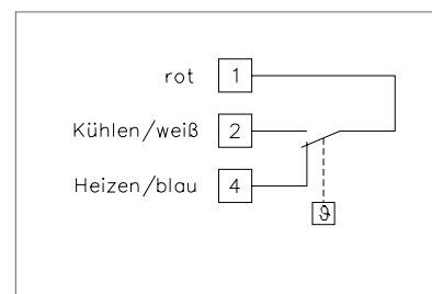
Anschlussbild TF einstufig
